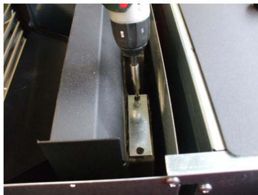
Fig. 44 - Rimozione tappi
