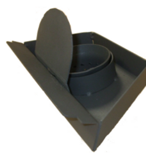
Fig. 35 - Posizione corretta del parafiamma
