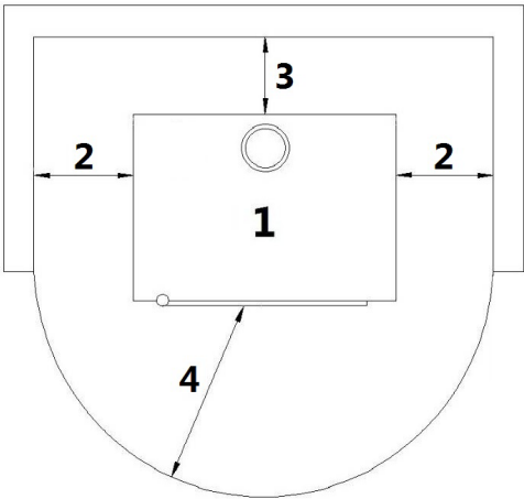
Fig. 12 - Installation générique
