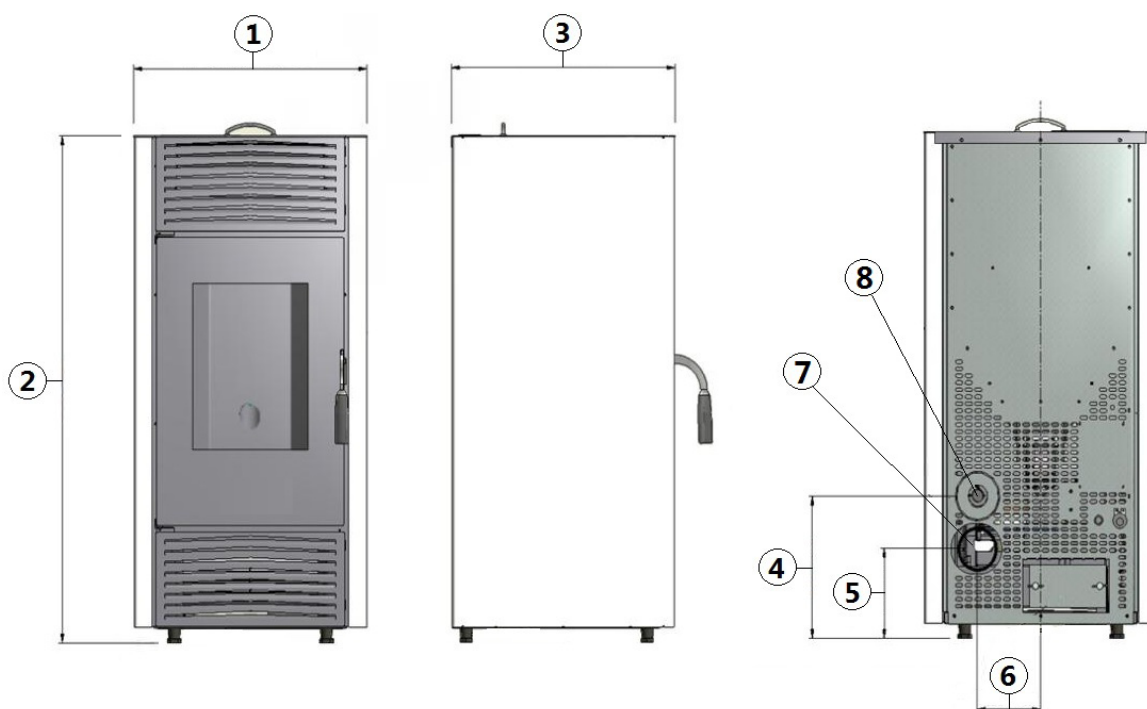
Fig. 11 - Dimensioni generali
