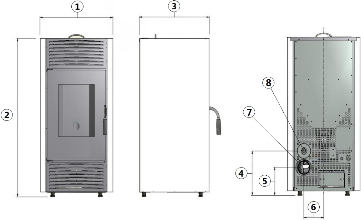
Fig. 11 - Dimensions générales
