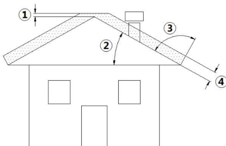
Fig. 2 - Tetto inclinato
