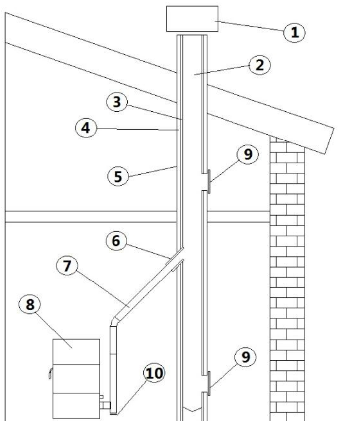
Fig. 5 - Componenti camino
