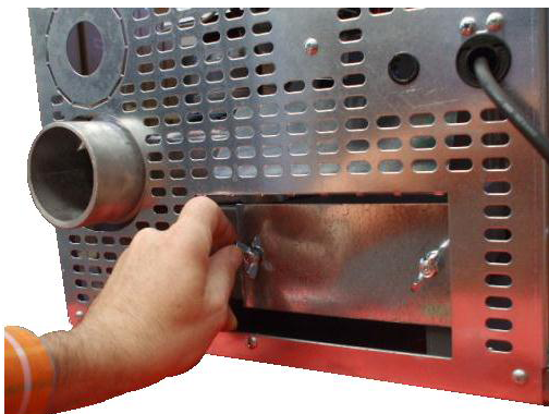
Fig. 37 - Chambre des fumées
