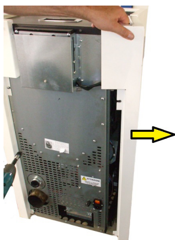
Fig. 19 - Aprire fianco
